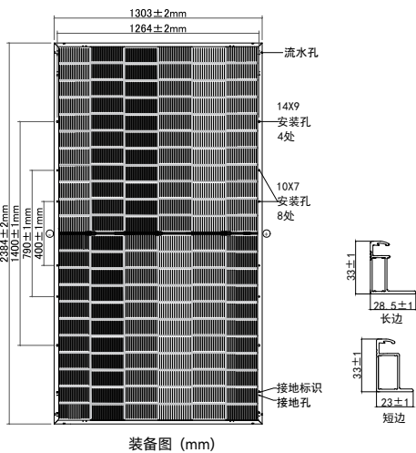
装备图 (mm)
